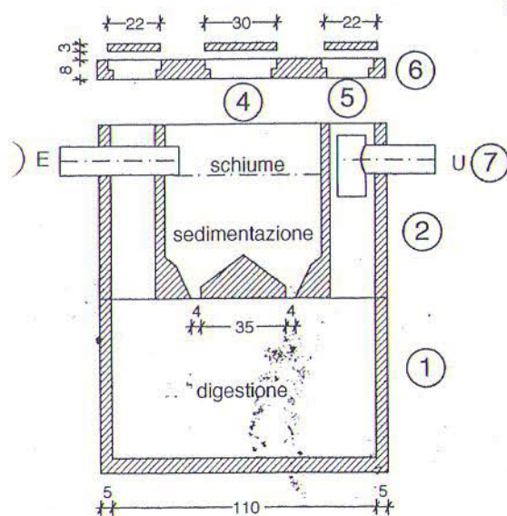
SEZ. B - B SCALA 1:20
